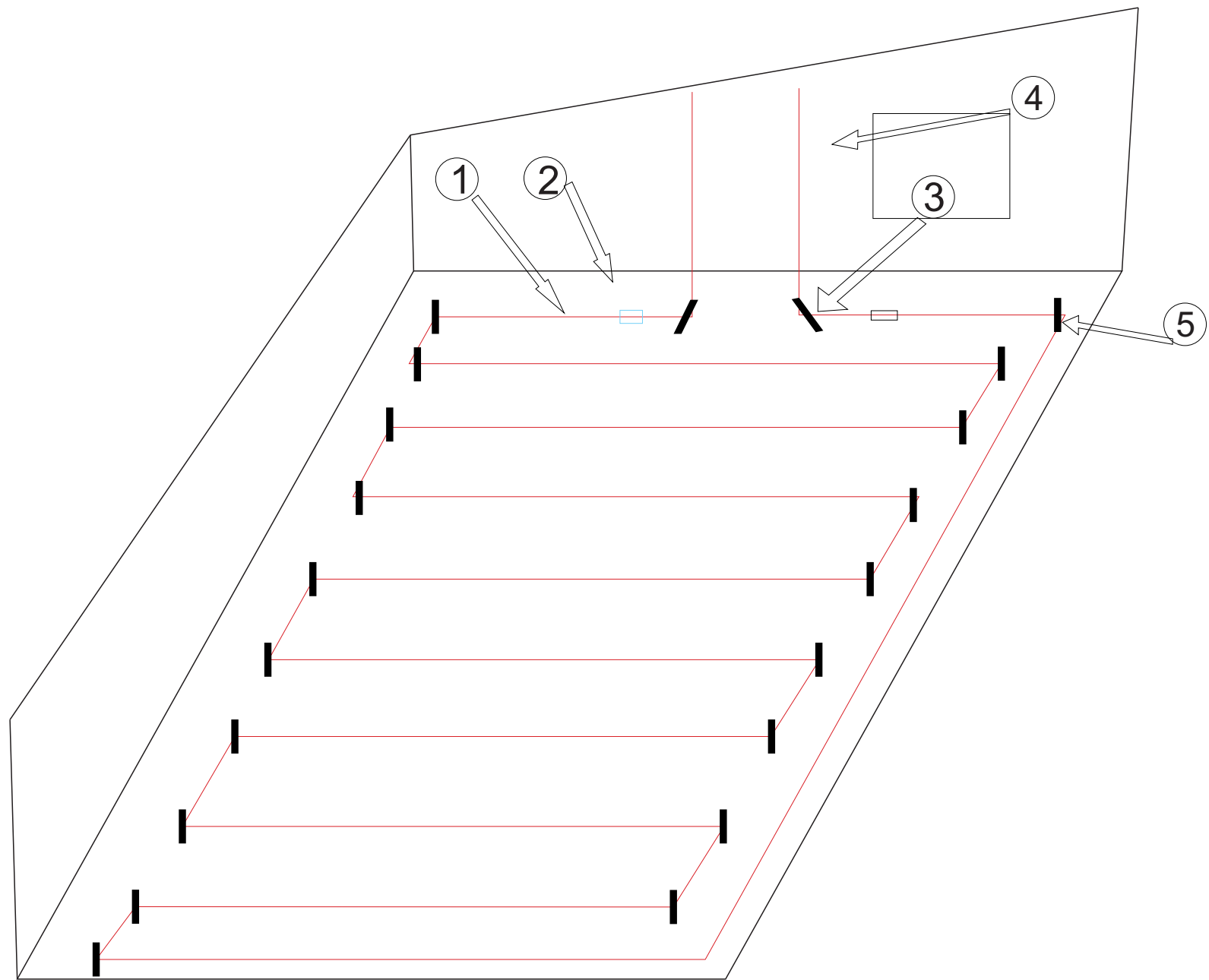
Šema postavljanja grejača
